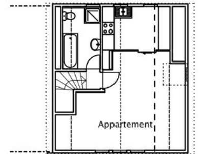
Obergeschoss
