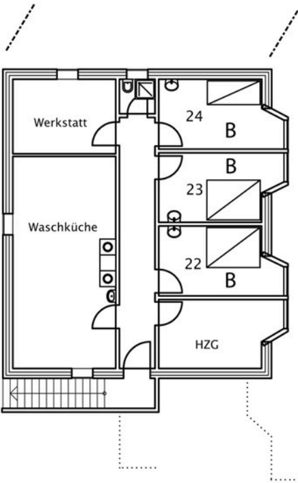
Tiefgeschoss
